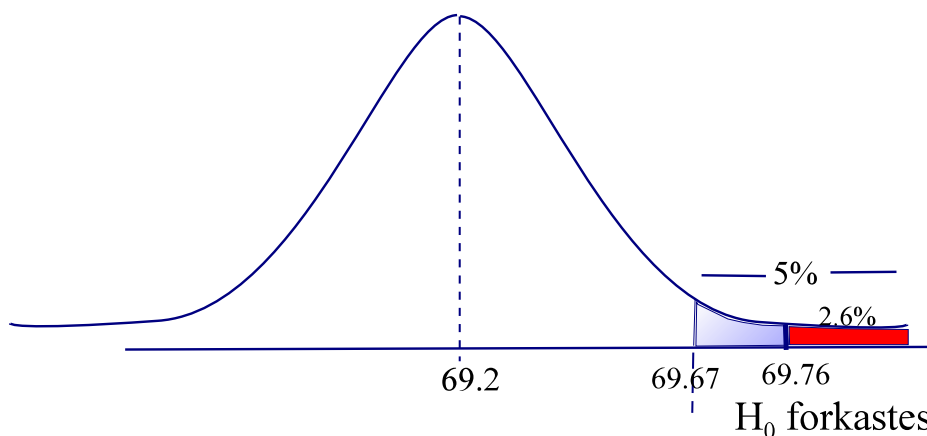
Fig 6.2 P-værdi
