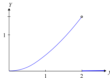
Fig.3.1 Tæthedsfunktion
